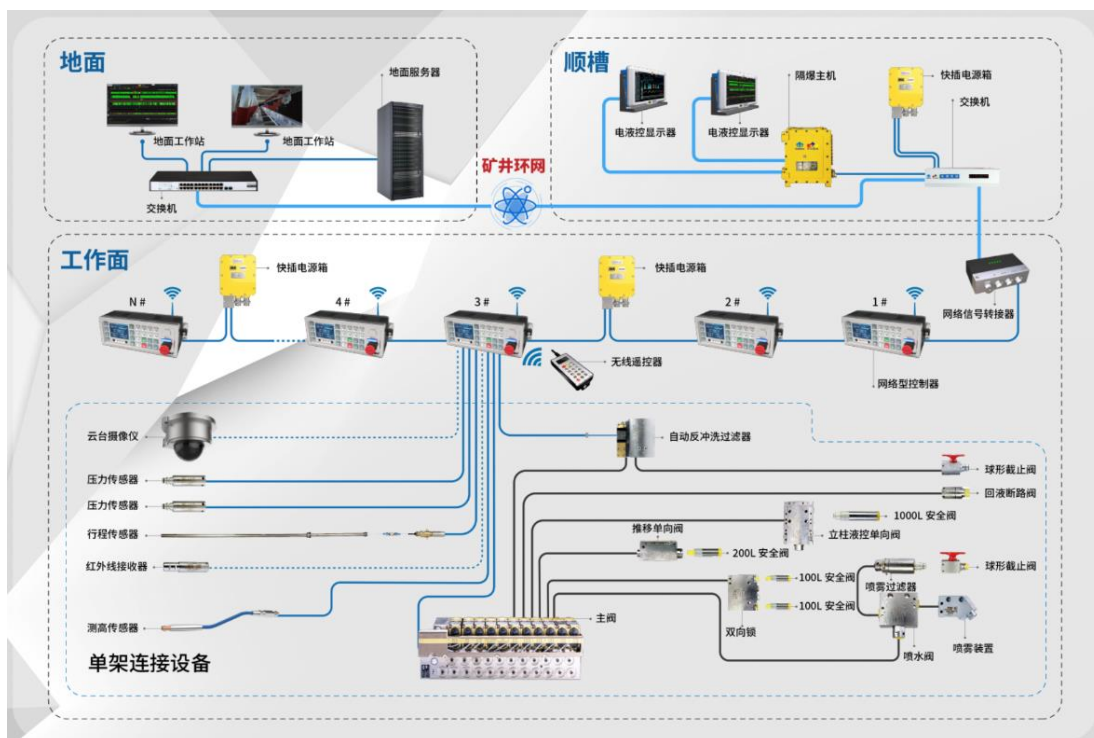
SAC 型液压支架电液控制系统
